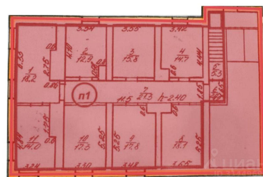
План цокольного этажа
